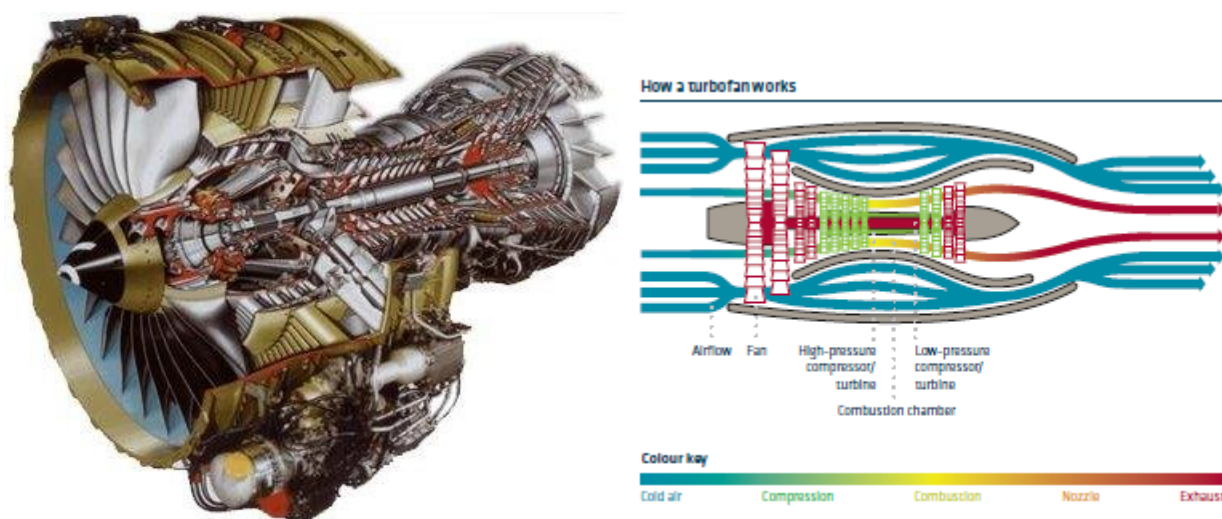
Figur 13 Medelstor jetmotor, CFM 56-7B, och principskiss
