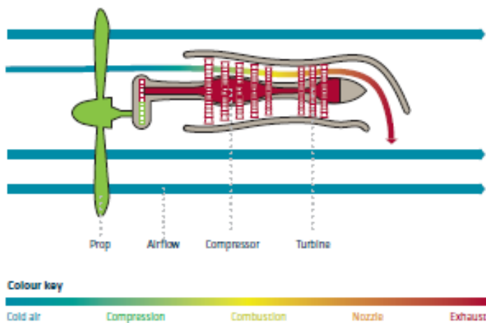
Figur 14 Principskiss för turbopropmotor
