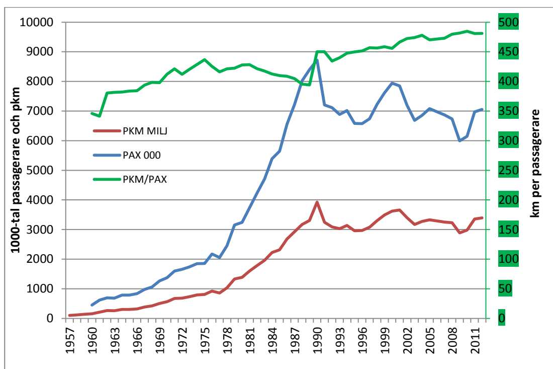
Figur 1 Inrikesflygets utveckling 1957-2012
